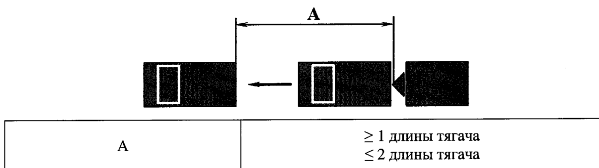
Рисунок 8. Схема и размеры маневра «Сцепление и расцепление или расцепление и повторное сцепление прицепа с тягачом (для транспортных средств категорий «BE», «CE» и «DE» и подкатегорий «C1E» и «D1E», за исключением сочлененных автобусов)» при расцеплении прицепа с тягачом
